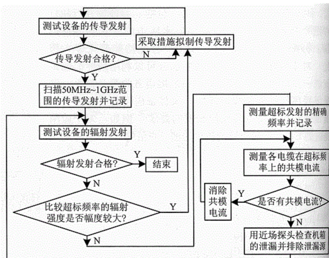
图1 电磁兼容测试诊断步骤
