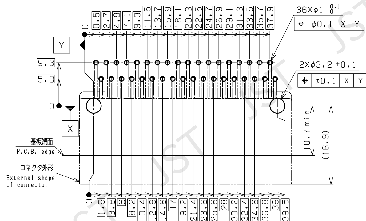
推奨パターンレイアウト／P.C.B. layout ＜コネクタ装着側／View from connector mounting side＞
