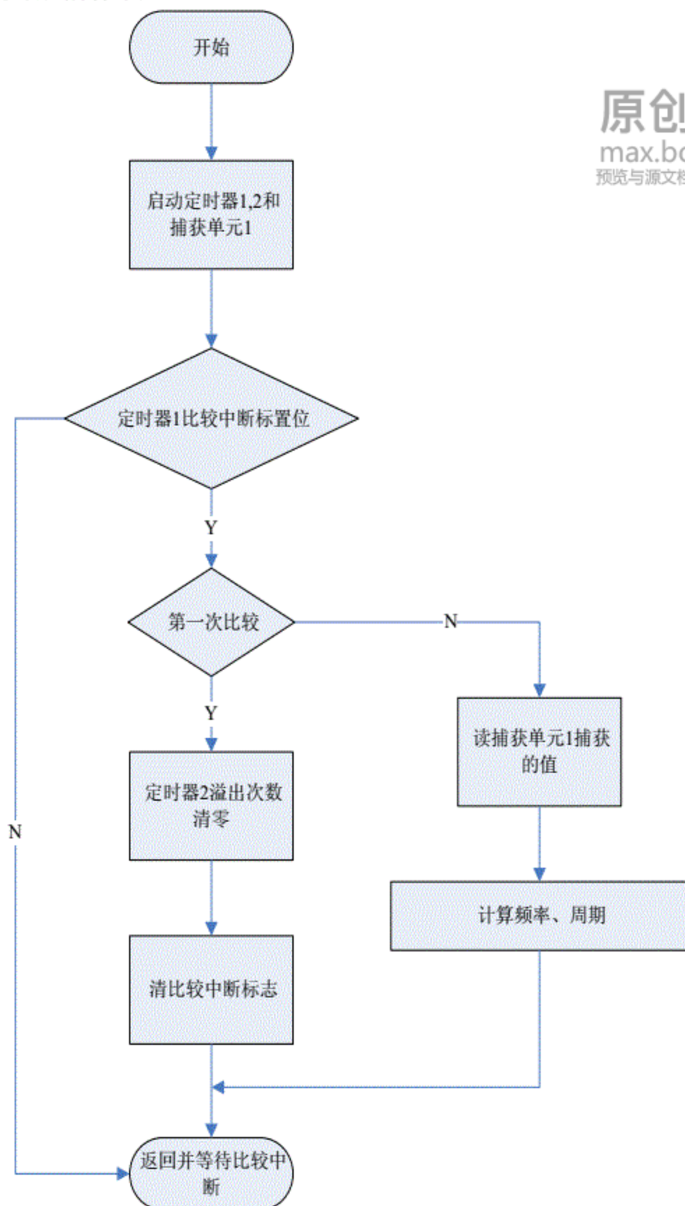
图9 定时器
