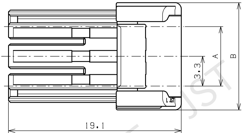
1 番極表示 No.1 Circuit Mark
