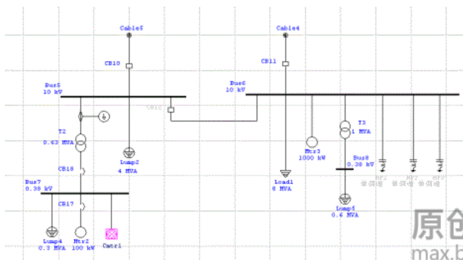
图 1-8 复合网络Network1的单线图
