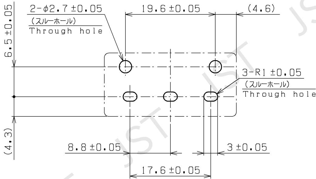
基板穴参考寸法 (コネクタ装着側より見る) Recommended P.C. Board Layout (View of component side)
