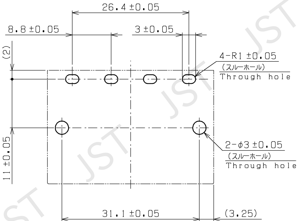
基板穴参考寸法 (コネクタ装着側より見る) Recommended P.C.Board Layout (View of component side)
