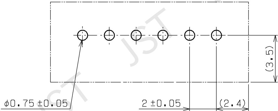
推奨基板穴寸法 (コネクタ装着側から見た図)
