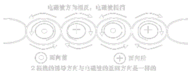
图7 绞线的抵消效果
