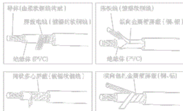
图5 屏蔽电线结构
