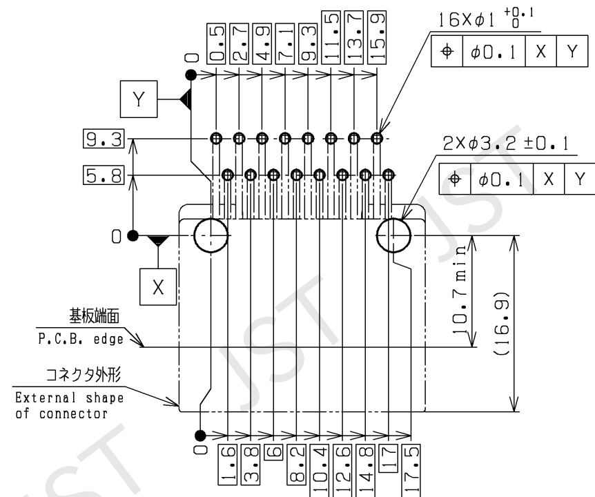
推奨パターンレイアウト / P.C.B. layout <コネクタ装着側 / View from connector mounting side>
