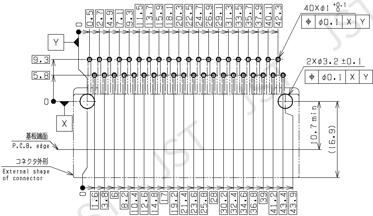
推奨パターンレイアウト／P.C.B. layout ＜コネクタ装着側／View from connector mounting side＞
