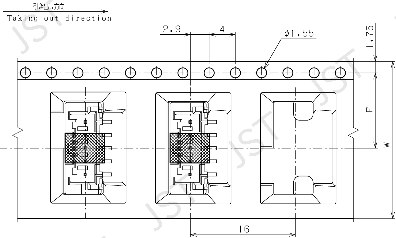
テープ幅W24のとき For the tape 24 in width
