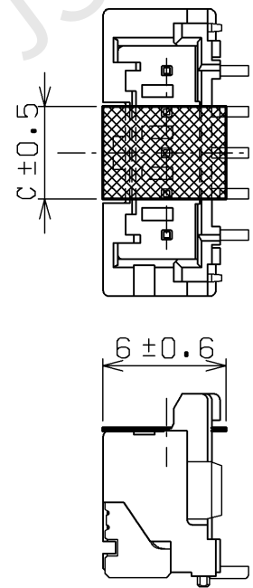
吸着テープ装着図 SUCTION TAPE CONFIGURATION
