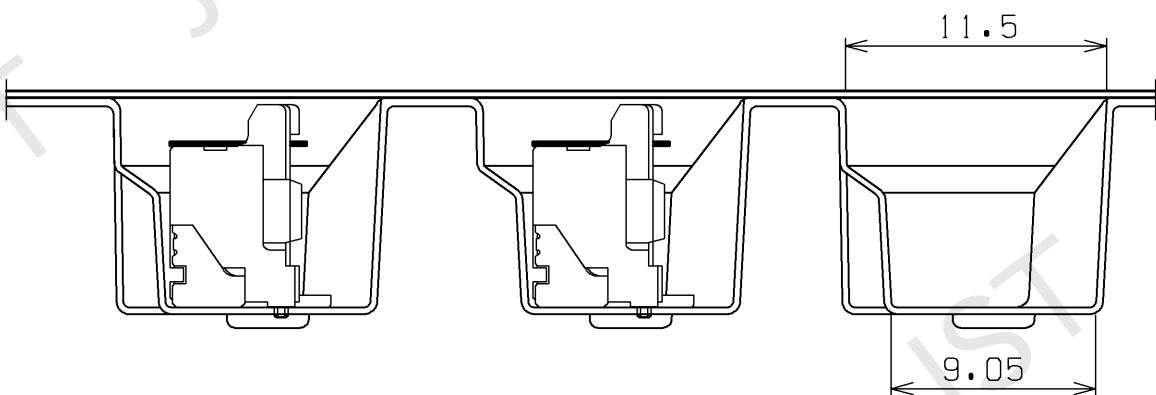
テープ幅W24のとき For the tape 24 in width
