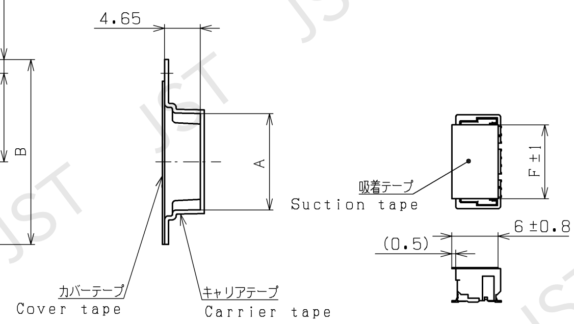
吸着テープ装着図 Configuration with suction tape
