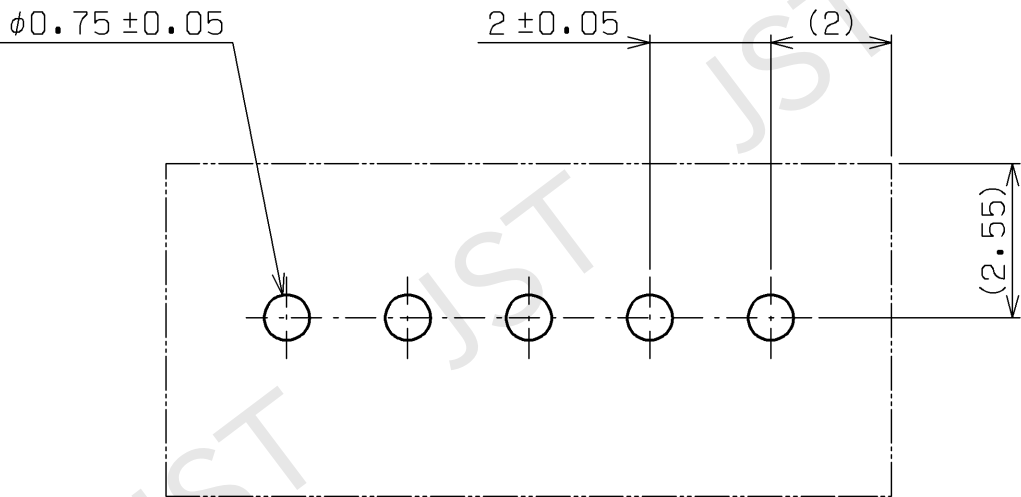
推奨基板穴寸法 (コネクタ装着側から見た図)
