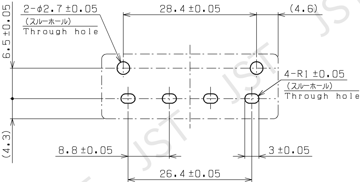
基板穴参考寸法 (コネクタ装着側より見る) Recommended P.C.Board Layout (View of component side)
