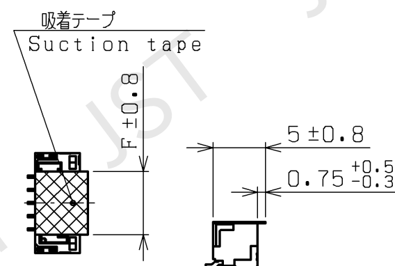
吸着テープ装着図 Suction tape configuration
