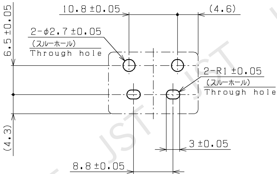
基板穴参考寸法 (コネクタ装着側より見る) Recommended P.C. Board Layout (View of component side)
