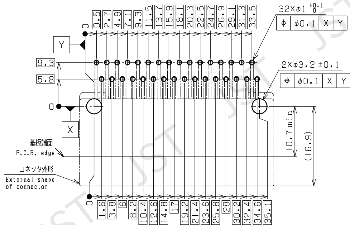
推奨パターンレイアウト/P.C.B. layout <コネクタ装着側/View from connector mounting side>
