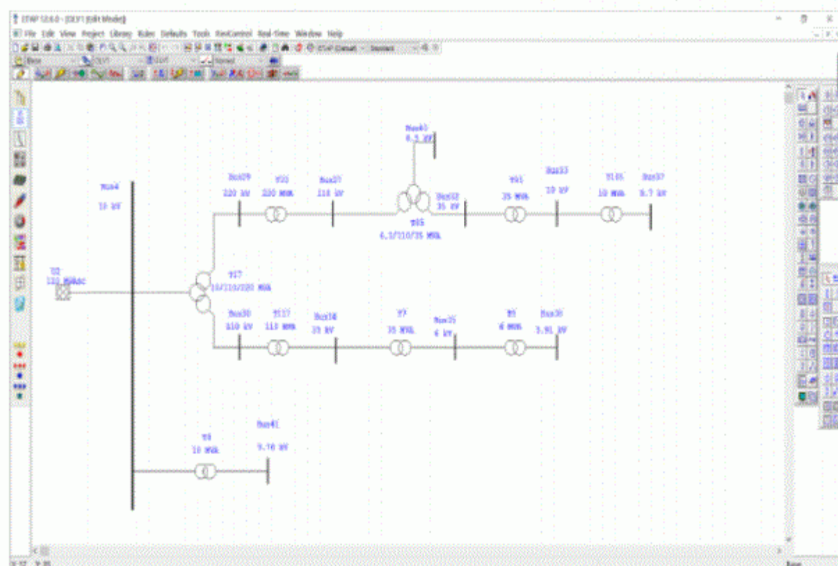
图 单线图
