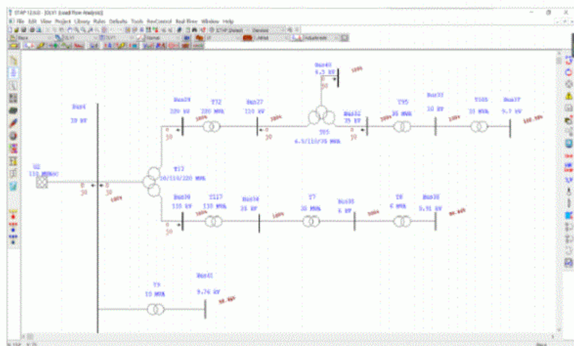
图 潮流分析计算后的单线图
