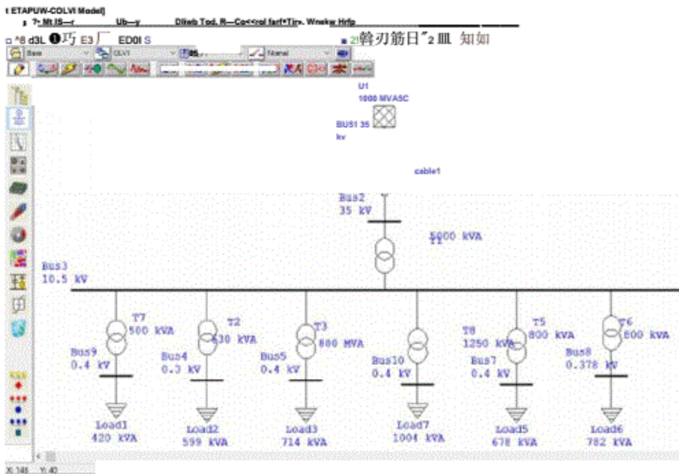
图 3.2 该报告单线图
