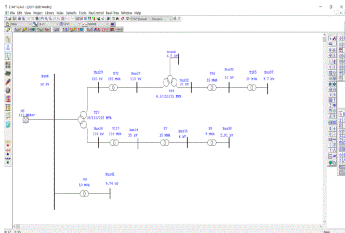
图3.3 单线图
