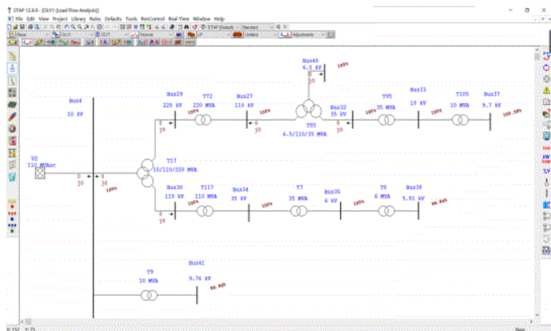
图 4.3 潮流分析计算后的单线图
