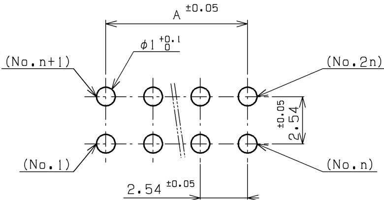
推奨基板レイアウト Recommendable P.C.Board layout
