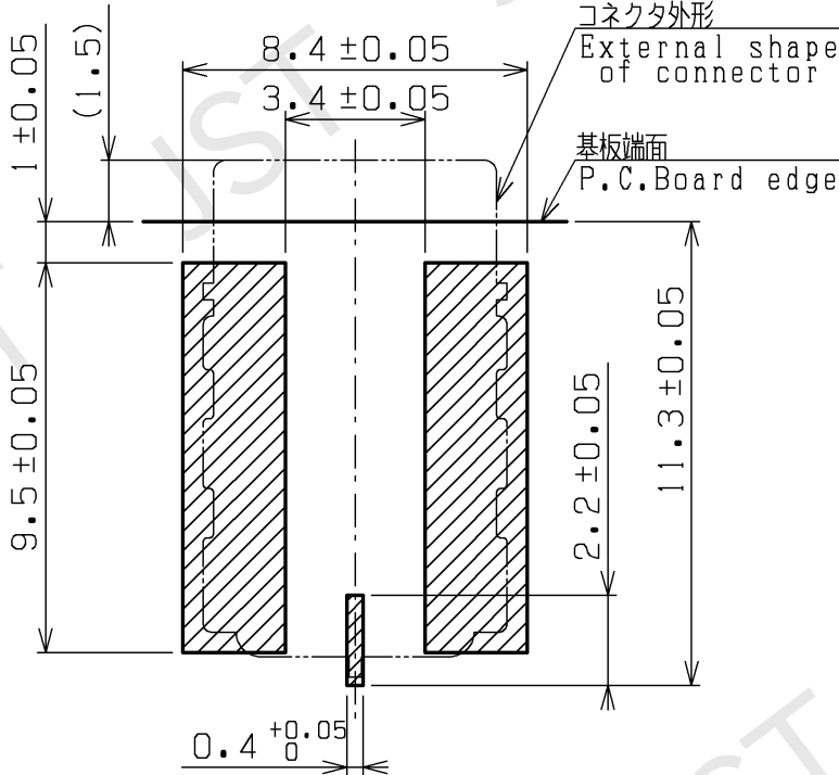
推奨基板レイアウト (参考) 部品搭載側 Recommendable P.C. Board layout (Reference) From top view
