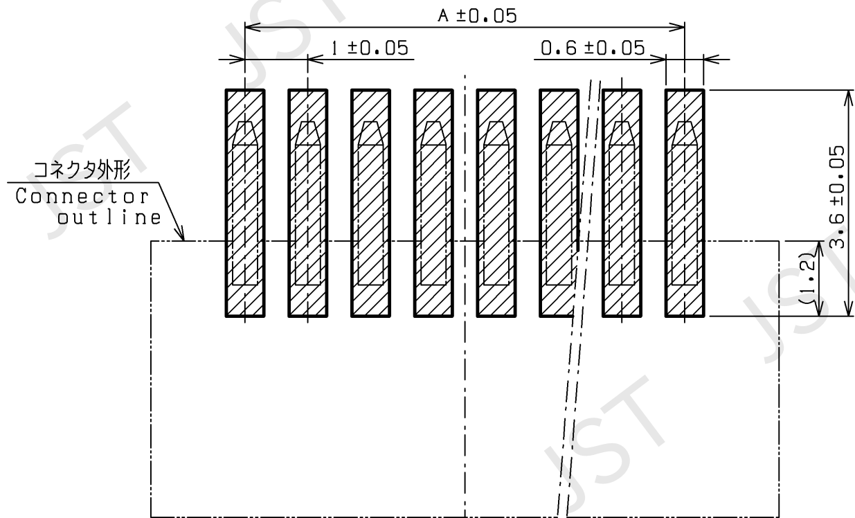
参考パターンレイアウト (コネクタ搭載面) Pattern layout (from top view)
