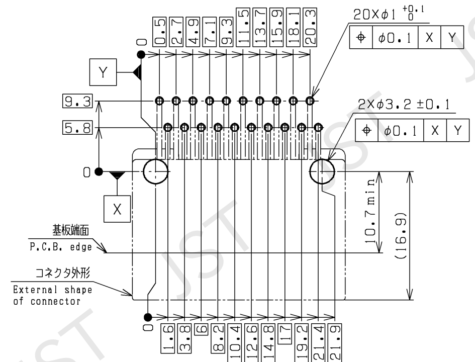
推奨パターンレイアウト / P.C.B. layout ＜コネクタ装着側 / View from connector mounting side＞
