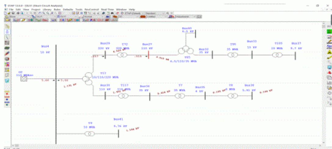
图4.7 三相短路计算后的单线图
