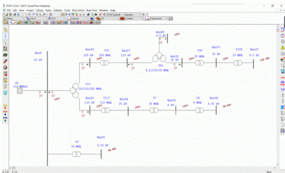
图 4.3 潮流分析计算后的单线图
