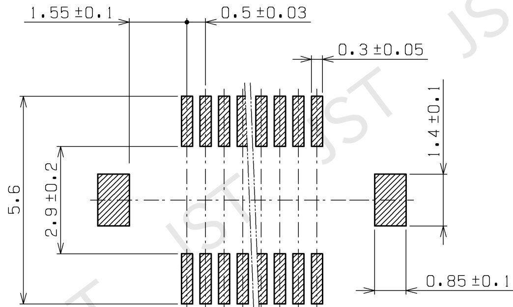
基板パターン推奨寸法 Recommendable P.C.Board layout
