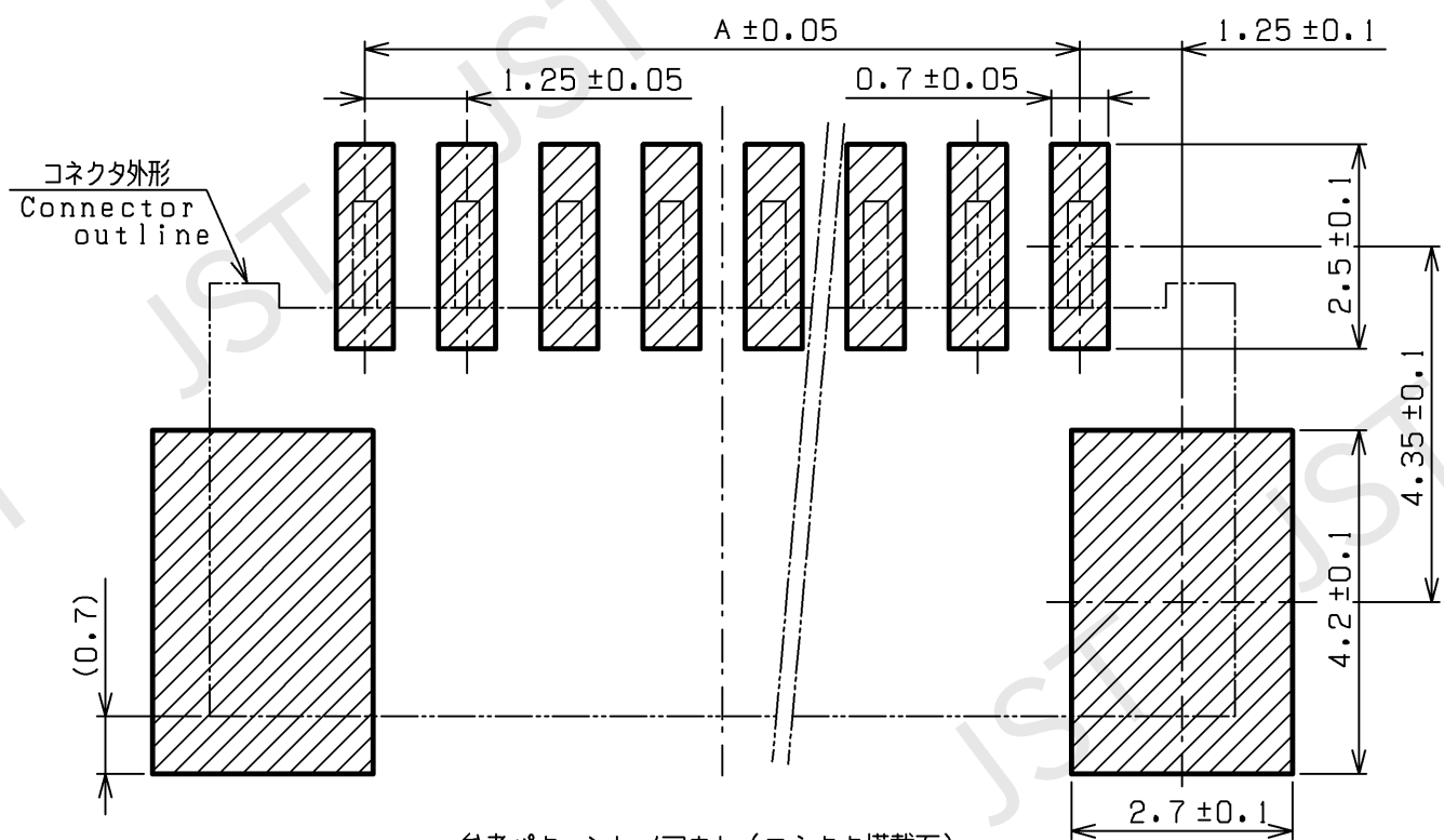
参考パターンレイアウト (コネクタ搭載面) Pattern layout (from top view)
