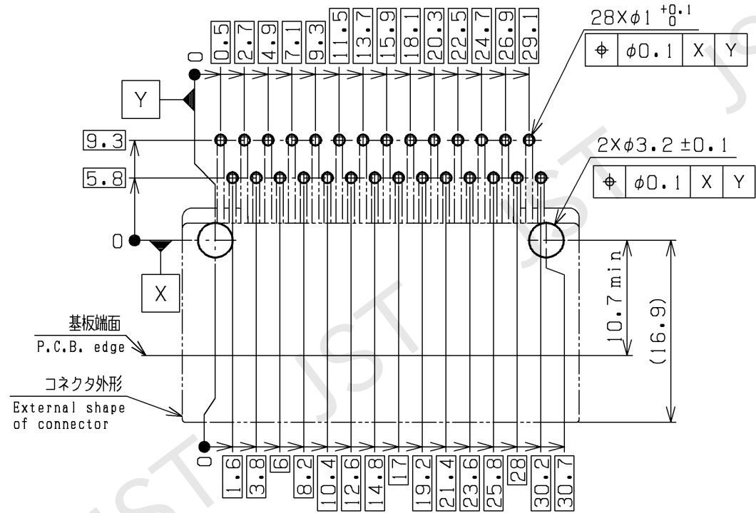
推奨パターンレイアウト / P.C.B. layout <コネクタ装着側 / View from connector mounting side>
