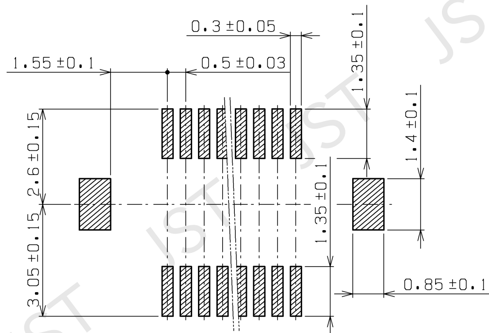
基板パターン推奨寸法 Recommendable P.C.Board layout
