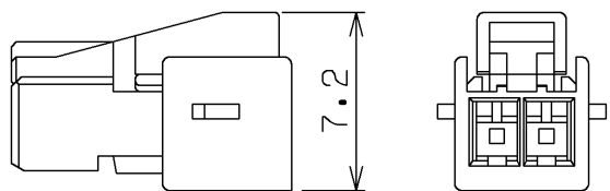
2極 (3:1) 2-circuits
