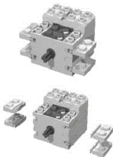
图 3.4 带有导轨的 1×2 的板便于固定马达
