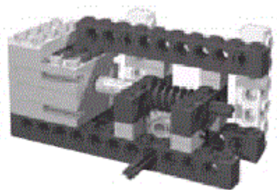
图 3.3 与蜗轮连接的马达
