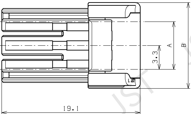
1 番極表示 No.1 Circuit Mark
