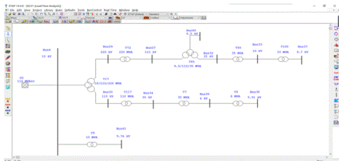
图4.1 潮流分析界面
