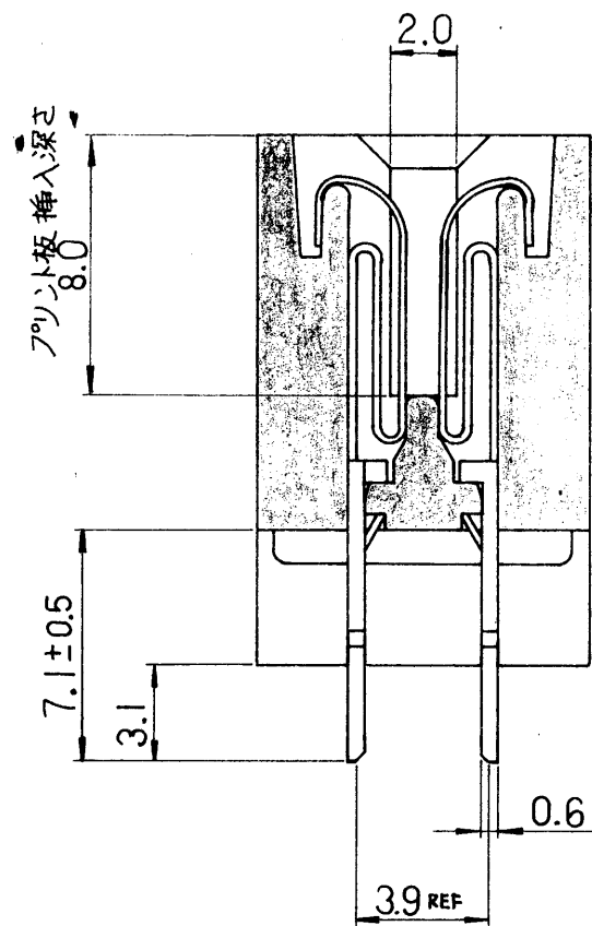
X-X'断面図 4/1
