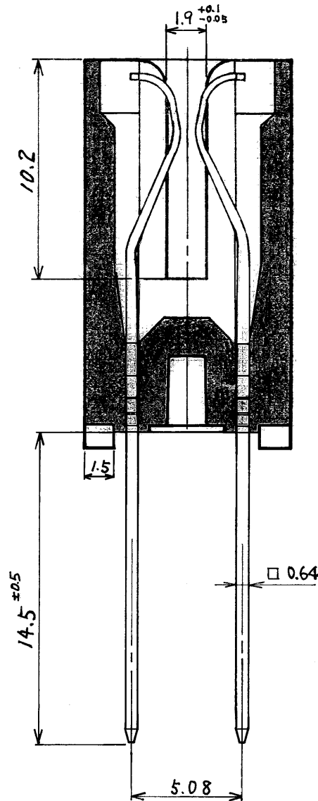
X-X' 断面图 尺度 4/1
