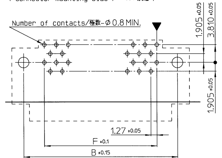
26・30・34・50 Pin
