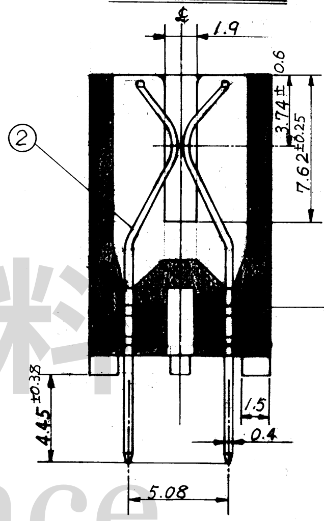
X-X'断面図 尺度 5/1
