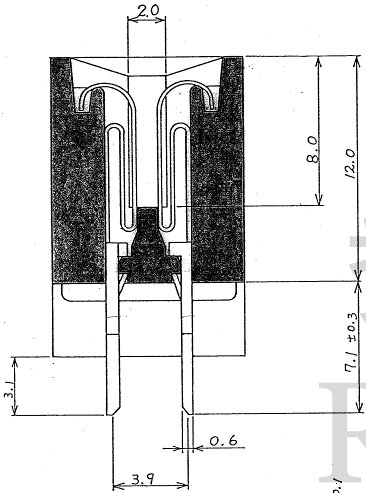
X-X'断面図 尺度 5/1
