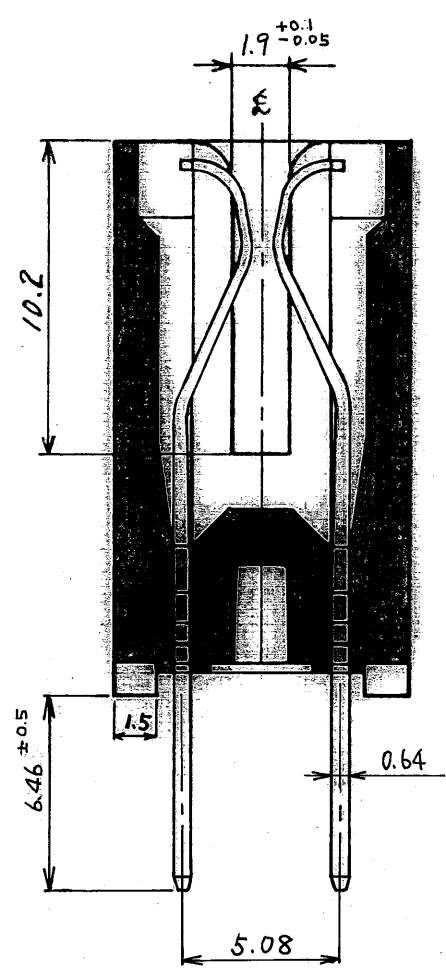
X-X' 断面図 尺度 4/1
