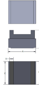
WCLA2520V1, WCLA3225V1
