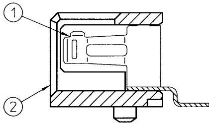
X-X'断面(5:1)
