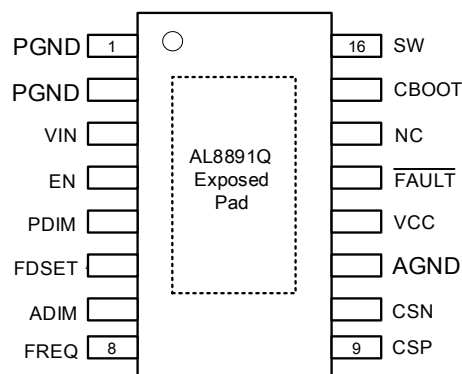
TSSOP-16EP
